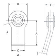
LIFT ARM END (BEND)
